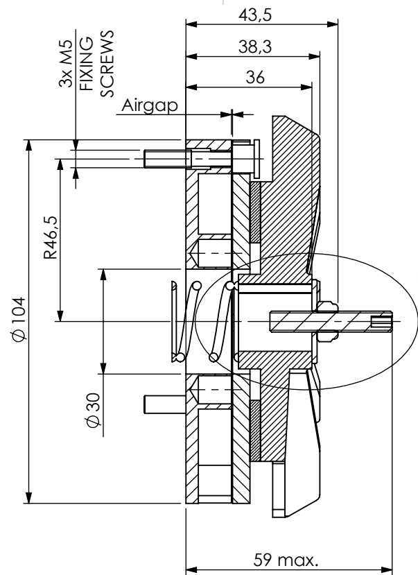
SEZIONE A-A
