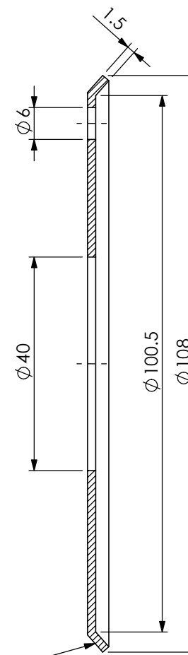
SEZIONE A-A
