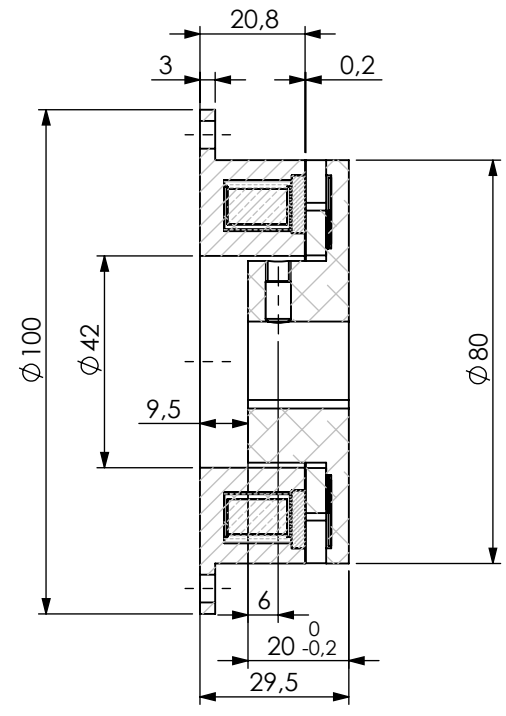
SECTION A-A SCALE 1 : 1.5
